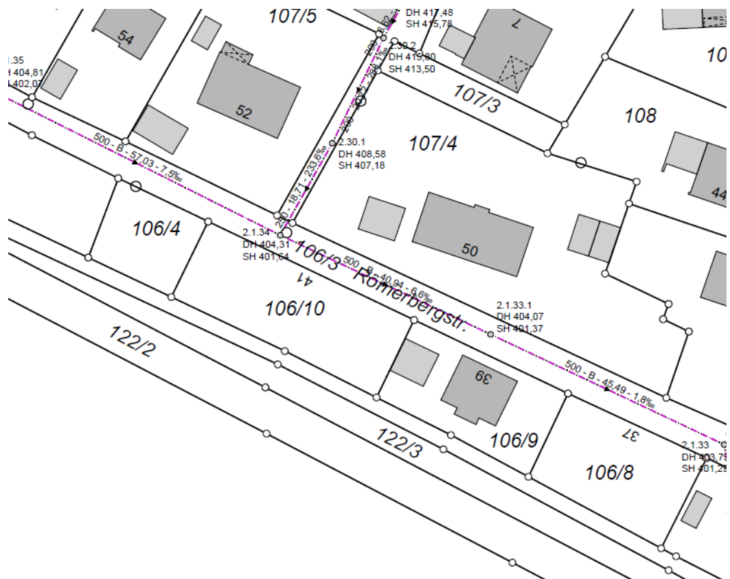
Bestandskanalplan
